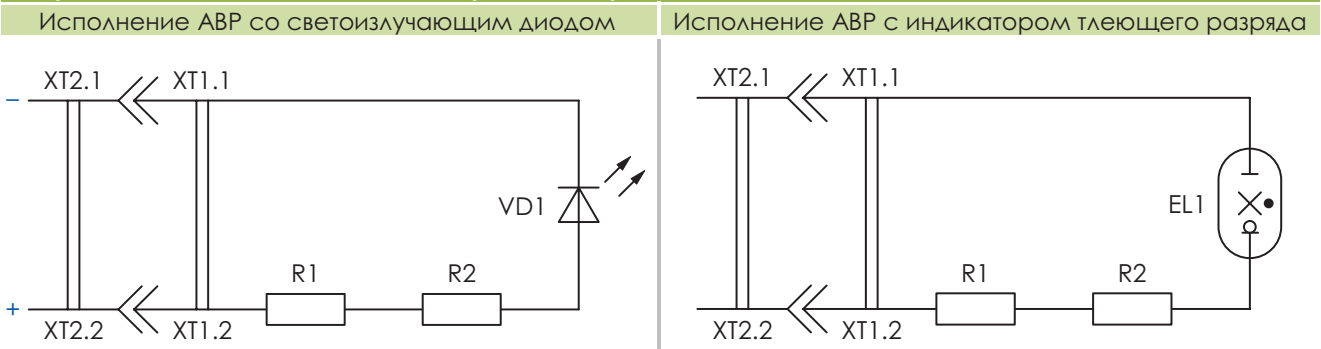
Рисунок 1 Схемы электрические принципиальные по исполнениям
