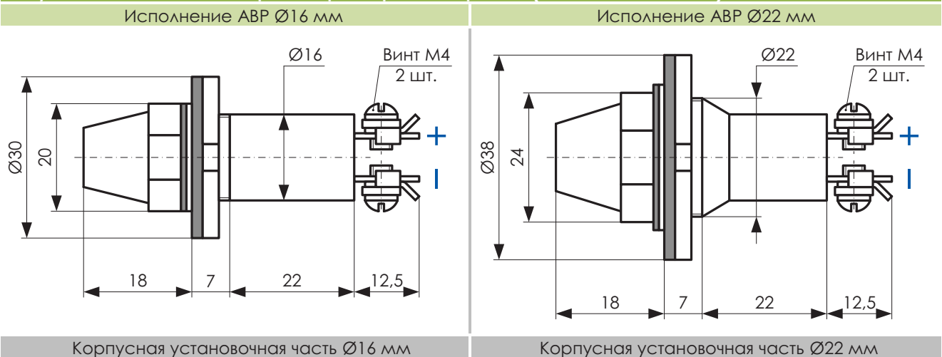
Рисунок 2 Габаритные размеры и полярность (на постоянном токе)
