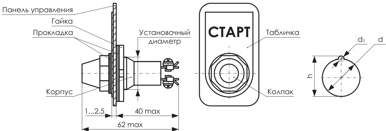
Рисунок 3 Установочные размеры, вариант монтажа и масса арматуры
